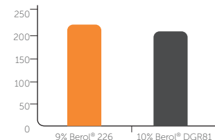
图3. 泡沫实验
